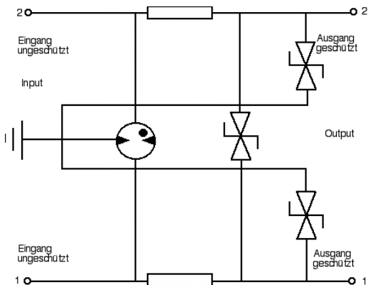
Innenschaltbild (Prinzip)
